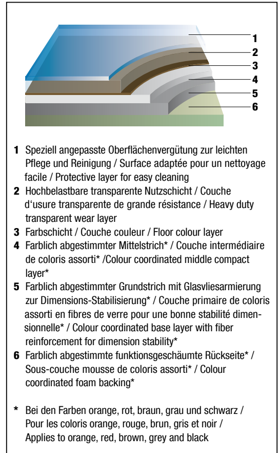
Bodenaufbau / Construction du tapis / Layer Structure
